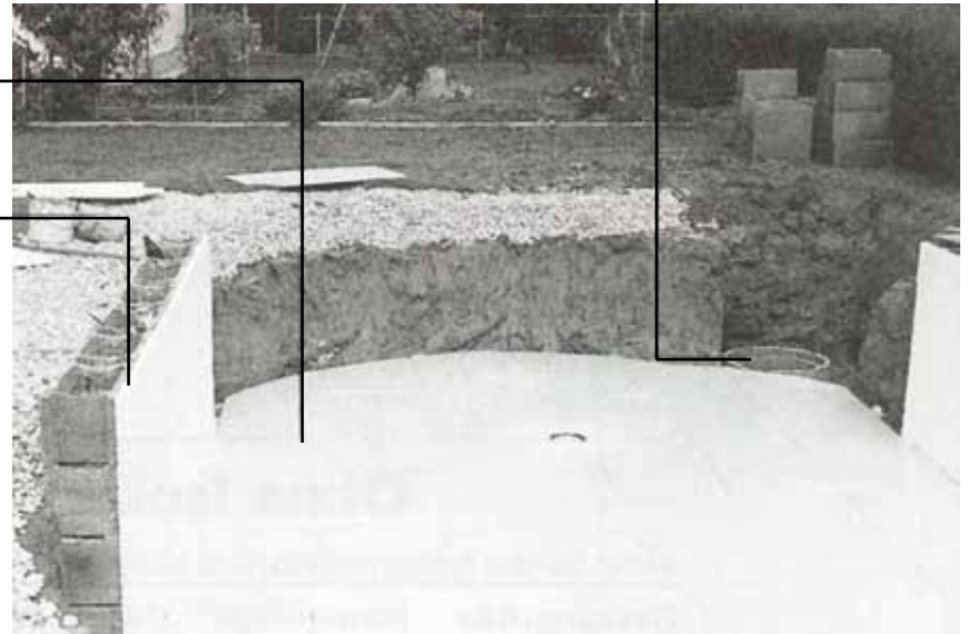
Sammelschacht für Ablauf
