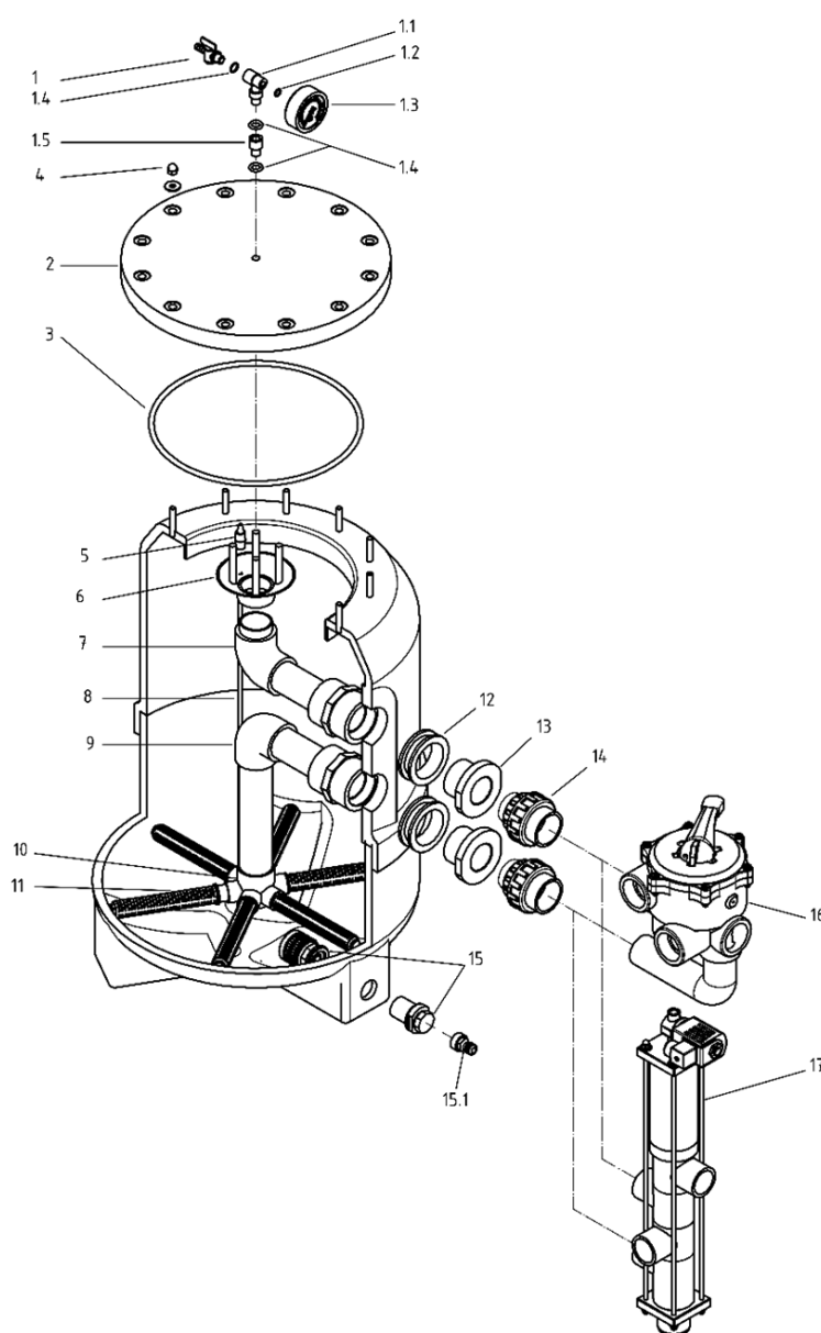
Abb. 3.1: DRESDEN 3 (ohne Pumpe dargestellt)
