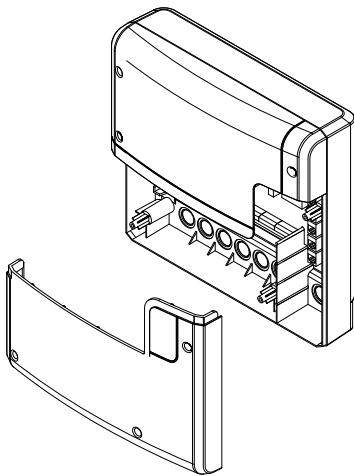
Leistungsteil, Unterteil der Frontabdeckung geöffnet
